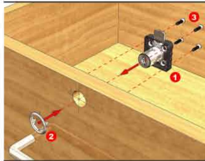
Mecanismo rectangular plástico Ø 17.5 mm 0201-088
