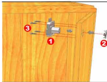
Mecanismo rectangular p/2 puertas Ø 17.5 mm 0201-089
