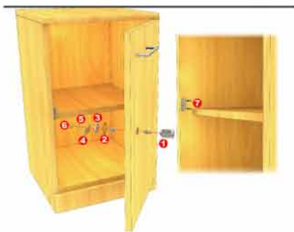
Mecanismo de paleta c/tuerca y arandela Ø 17.5mm 0201-098
